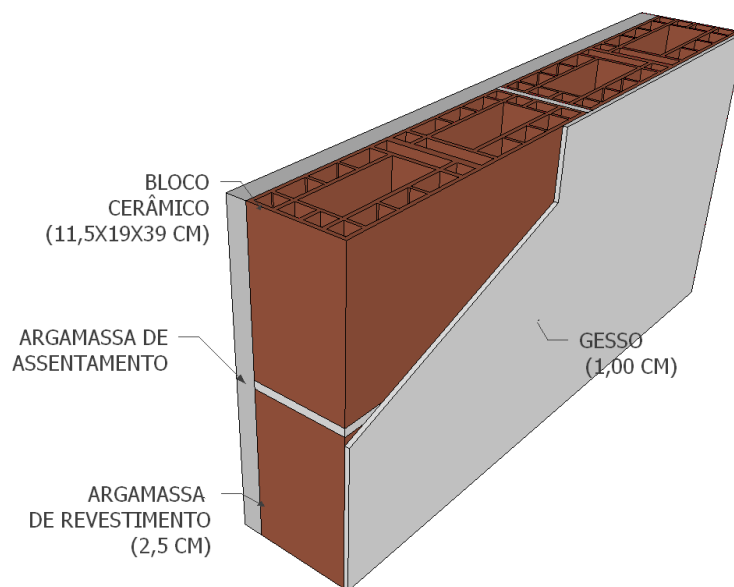
Figura 1 - Esquema do elemento construtivo, objeto dessa FAD
