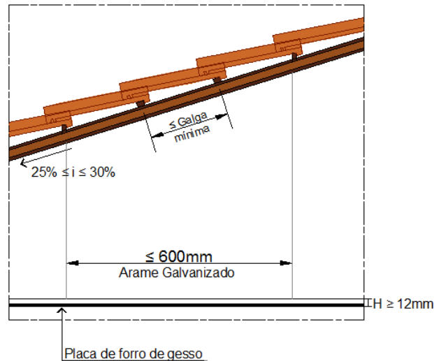
Figura 1 - Sistema de cobertura composto por telha cerâmica simples de sobreposição modelo Colonial, estrutura de madeira e forro de gesso
