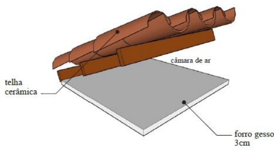
Figura 17 - Propriedades térmicas do sistema de cobertura (Fonte: Anexo Geral V – Catálogo de Propriedades Térmicas de Paredes, Coberturas e Vidros – Anexo da Portaria do INMETRO Nº50/2013)
