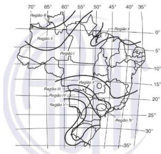
Figura 16 – Condições de exposição de acordo com as regiões do Brasil (ABNT NBR 6123:1988/Er2:2013)
