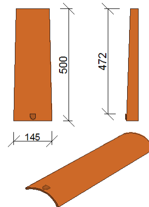
Figura 2 – Características dimensionais da telha cerâmica simples, modelo Colonial
