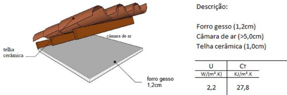
Figura 18 - Propriedades térmicas do sistema de cobertura objeto da FAD
