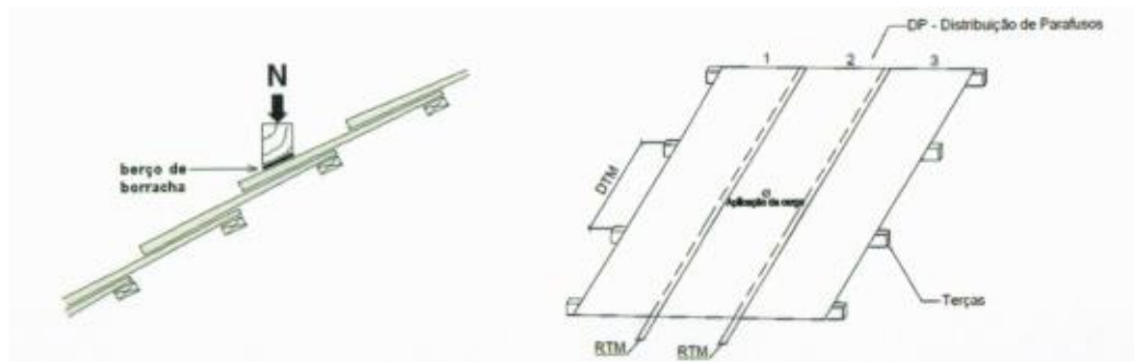
Figura 13 – Carga concentrada transmitida com o auxílio de cutelo de madeira e berço de borracha
