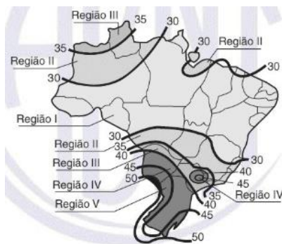
Figura 10 – Gráfico das isopletas da velocidade básica do vento, “ V_0 ”, em metros por segundo, no Brasil (ABNT NBR 6123:1988/Er2:2013)
