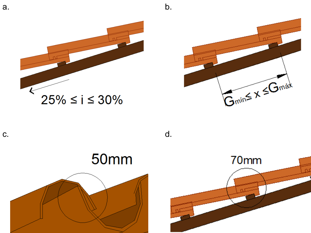
Figura 4 – Orientações para montagem do telhado
